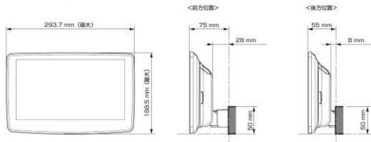
ディスプレイユニット寸法
