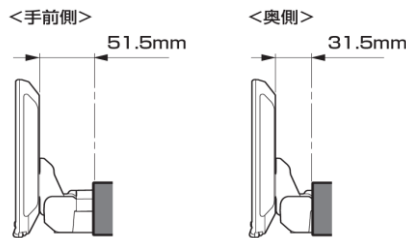
【ディスプレイユニット前後位置】
