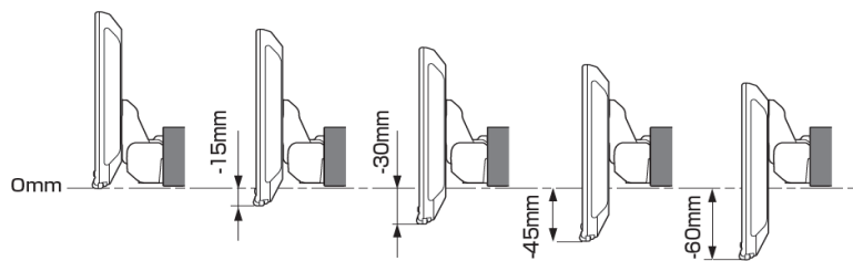
【ディスプレイユニット上下位置】
