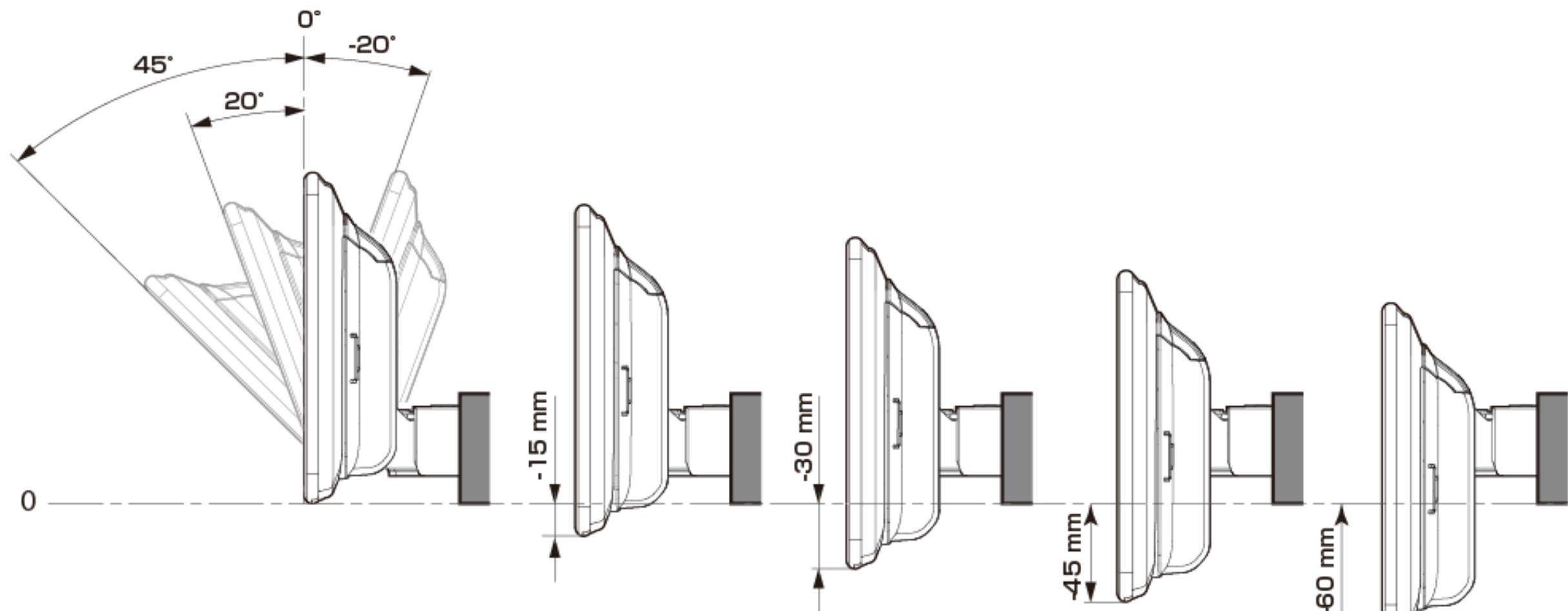
調整可能なディスプレイ角度および上下の位置
