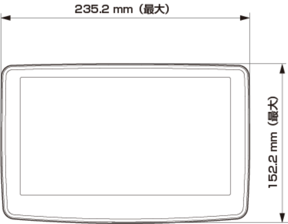
ディスプレイユニット寸法
