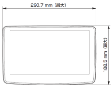
■ ディスプレイ取り付け寸法と調整可能位置
