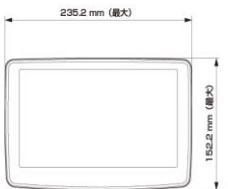
ディスプレイユニット寸法
